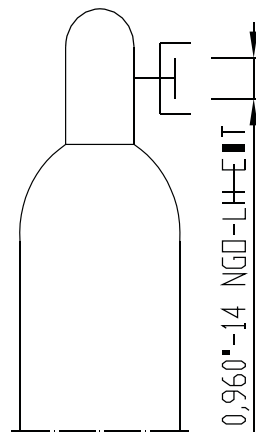
美式 SF 6 气瓶
