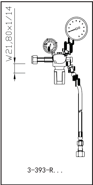
适配的连接部件
