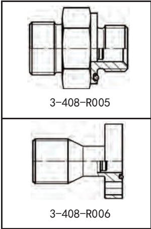
适配的连接部件
