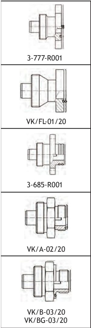
适配的连接部件
