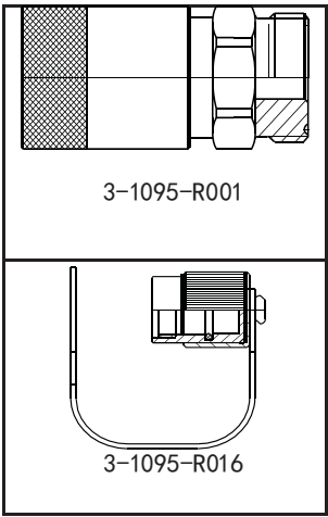
适配的连接部件
