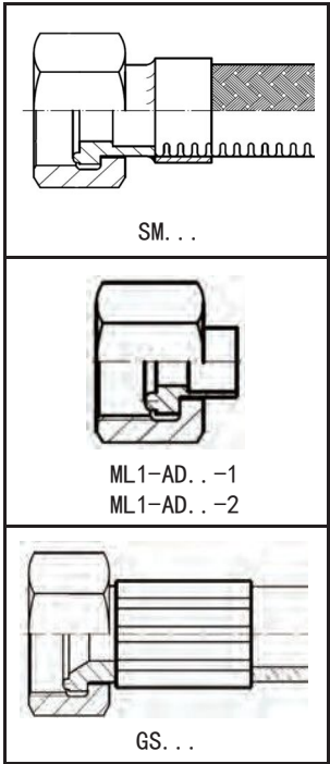
适配的连接部件
