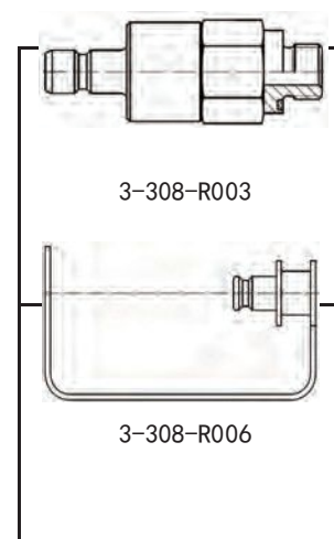
适配的连接件
