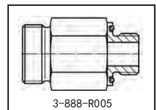
适配的连接部件
