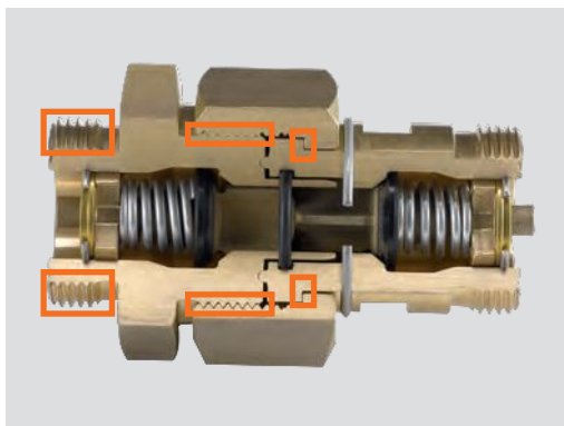
10. DIL0 管道连接件的润滑点
